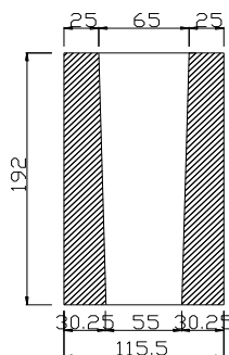
SEZIONE A-A
