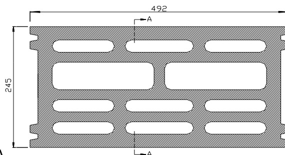
PIANTA
