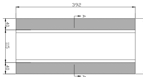
PIANTA
