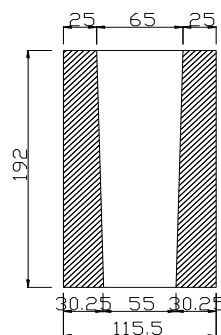
SEZIONE A-A
