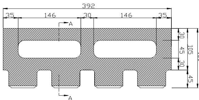
PIANTA
