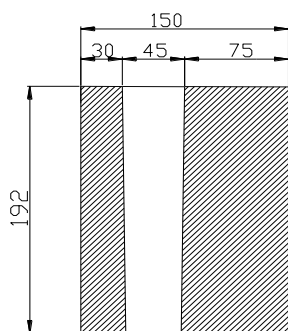
SEZIONE A-A
