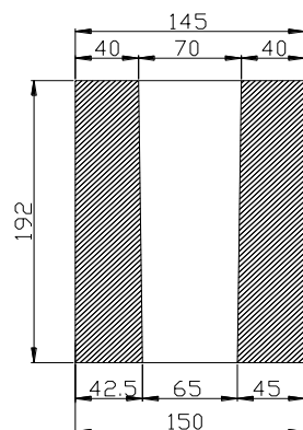
SEZIONE
