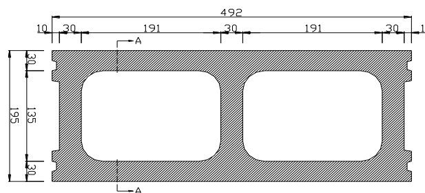
PIANTA
