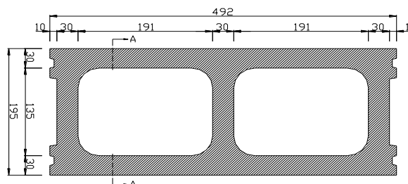
PIANTA
