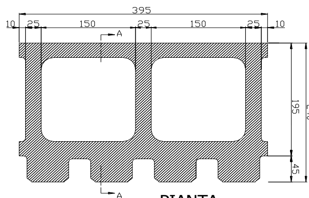
PIANTA
